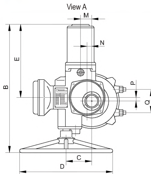
Type 9034/4027
