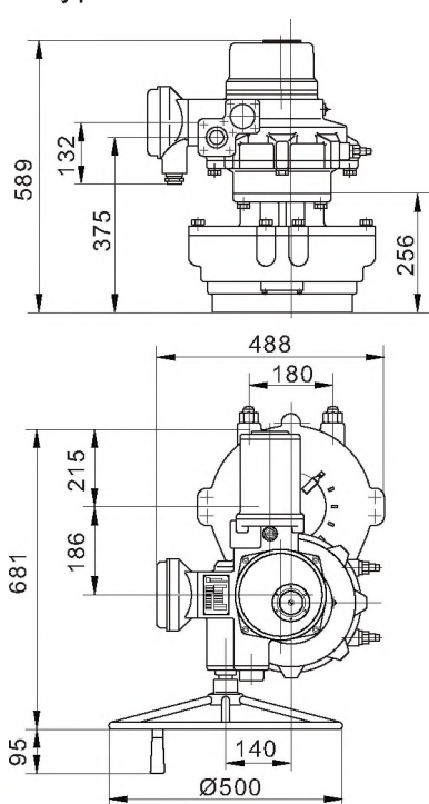
Type 802. 1000-0. 2
