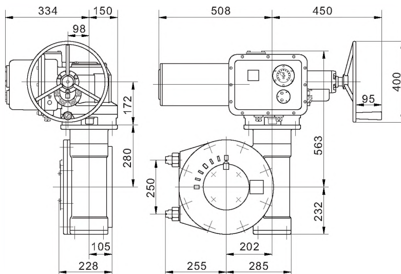
Type 9034/4027
